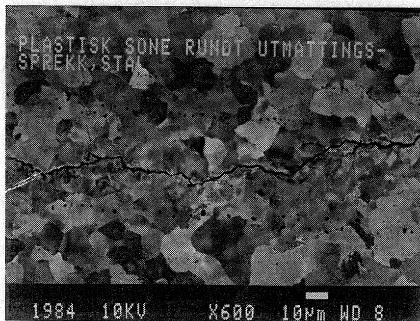
Fig. 60. Plastisk deformasjonssone rundt en utmattingssprekk i stål.
