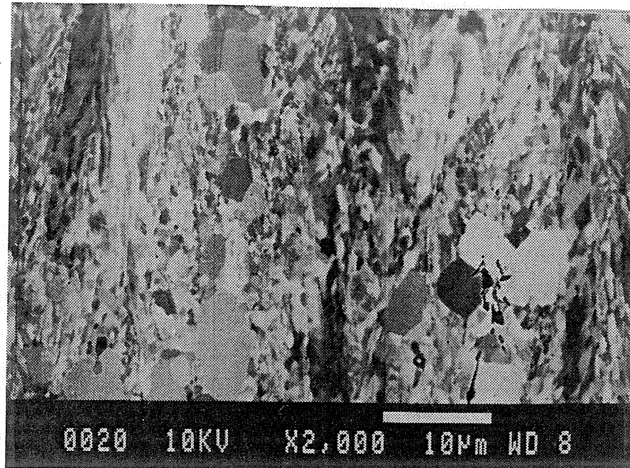
Fig. 59. Delvis rekrySTALLisert stålprøve.
