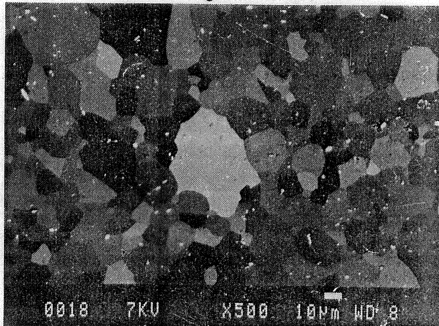
Fig. 57. Diffraksjonskontrast fra Al-legering.
