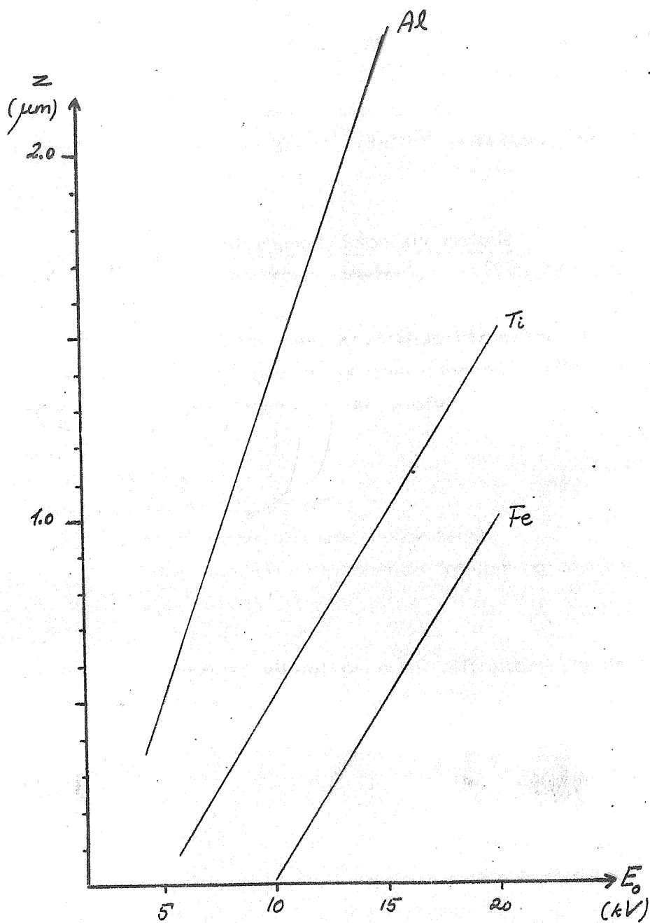
Fig. 41. Emisjonsdybde for karakteristisk K-røntgenstråling for elementene Al, Ti og Fe som funksjon av akselerasjons-spennning.
