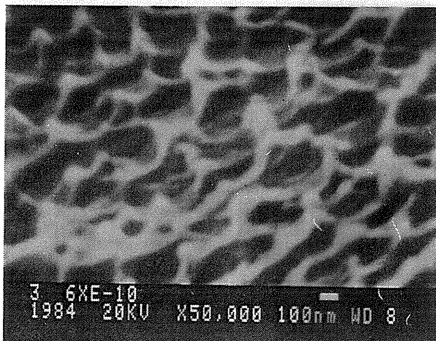
Fig. 17. Opplysningen er betydelig forbedret ved at strømmen i primærstrålen er redusert til 6 \times 10^{-10} A.
