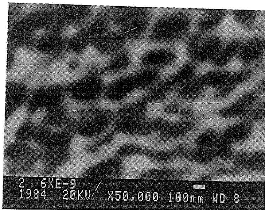
Fig. 16. Uskarpt bilde p.g.a. høy strøm i primærstrålen, i = 6 \times 10^{-9} A.
