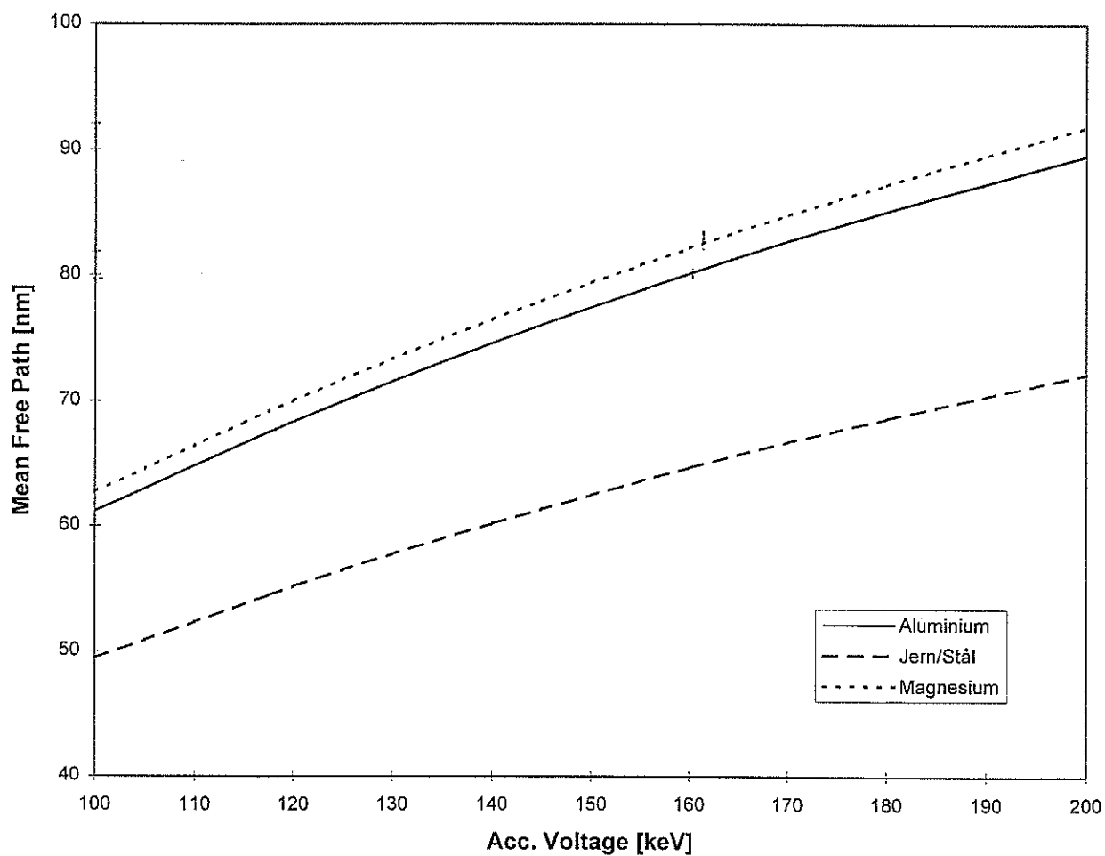
Midlere fri veilengde for aluminium, magnesium og jern/stål (Beta=100 mrad)
