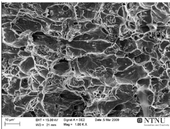
Ductile Fracture with dimples Duktilt brudd med krusninger
